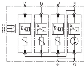
Schemat połączeń DG M TT 150 FM
