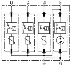
Schemat połączeń DG M TT 385
