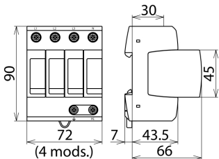
Rysunek wymiarowy DG M TT 385
