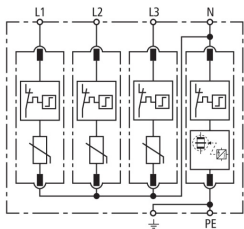
Schemat połączeń DG M H TT 275
