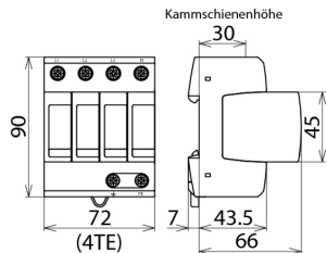
Rysunek wymiarowy DG M H TT 275
