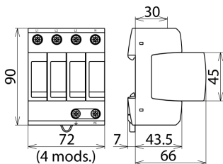
Rysunek wymiarowy DG M TNS 385
