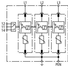
Schemat połączeń DG M TNC 150 FM
