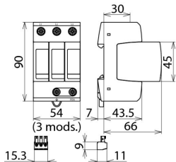
Rysunek wymiarowy DG M TNC 150 FM
