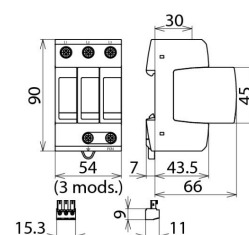
Rysunek wymiarowy DG MP WE 600 FM
