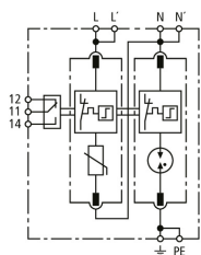
Schemat połączeń DG MP TT 2P 275 FM
