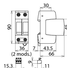
Rysunek wymiarowy DG MP TT 2P 275 FM
