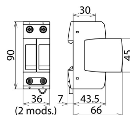
Rysunek wymiarowy DG MP TN 150 FM
