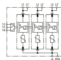
Schemat połączeń DG MP TNC 275 FM
