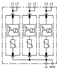
Schemat połączeń DG MP TNC 275 FM
