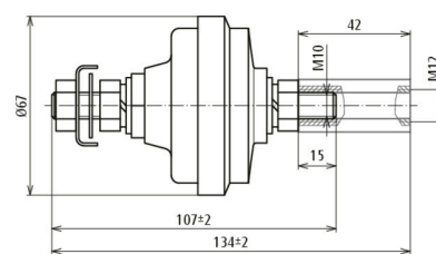
Rysunek wymiarowy DIC 10
