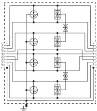
Schemat połączeń DPA CLE IP66
