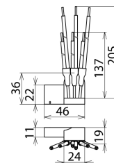
Rysunek wymiarowy DFL D 255
