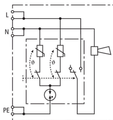
Schemat połączeń DFL D 255
