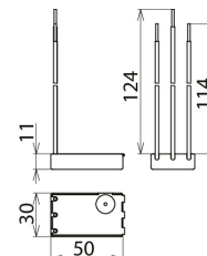
Rysunek wymiarowy DFL M 255
