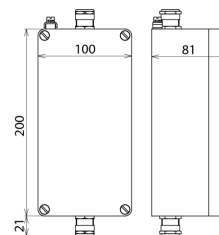
Rysunek wymiarowy ALGA 5
