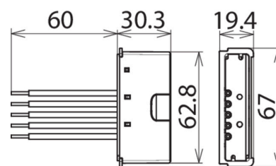
Rysunek wymiarowy DCOR L 3P 275 SO LTG
