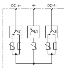
Schemat połączeń DG YPV SCI 600
