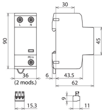
Rysunek wymiarowy DSH B TT 2P 255 FM
