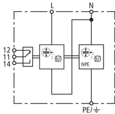
Schemat połączeń DSH B TT 2P 255 FM
