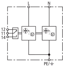
Schemat połączeń DSH B TN 255 FM
