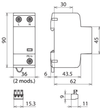
Rysunek wymiarowy DSH B TN 255 FM
