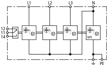
Schemat połączeń DSH TT 255 FM
