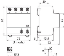
Rysunek wymiarowy DSH TT 255 FM
