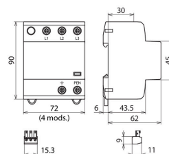
Rysunek wymiarowy DSH TNC 255 FM
