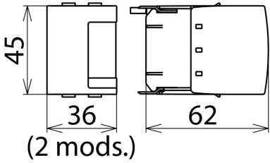
Rysunek wymiarowy DV MOD NPE 50
