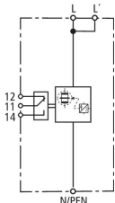
Schemat połączeń DBM 1 440 FM
