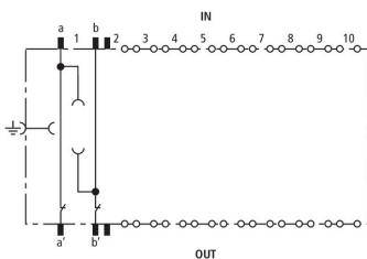
Schemat połączeń BM 10 DRL
