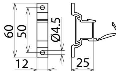
Rysunek wymiarowy SH 18X3 K
