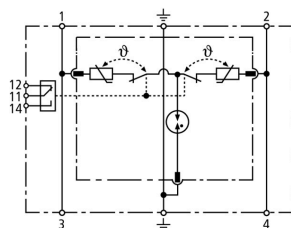
Schemat połączeń DR M 2P 150 FM
