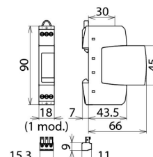
Rysunek wymiarowy DR M 2P 75 FM
