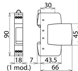
Rysunek wymiarowy DR M 2P 75
