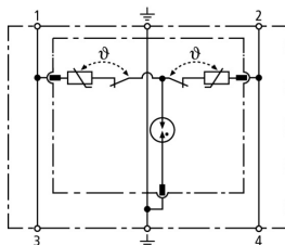
Schemat połączeń DR M 2P 75
