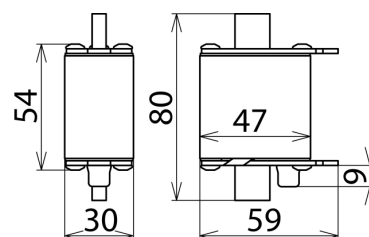
Rysunek wymiarowy VA NH00 280
