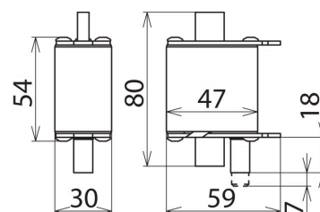
Rysunek wymiarowy V NH00 280 FM
