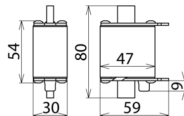
Rysunek wymiarowy V NH00 280
