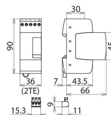
Rysunek wymiarowy DR M 4P 255 SN1872 FM
