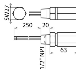
Rysunek wymiarowy DPI CD EXD 230 24 N
