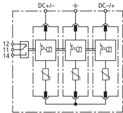
Schemat połączeń DG M YPV 1200 FM
