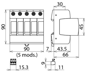
Rysunek wymiarowy DG M PV2 SCI 1000 FM
