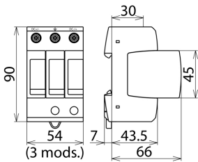
Rysunek wymiarowy DG M YPV SCI 1200
