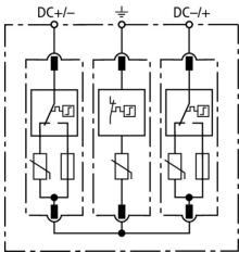
Schemat połączeń DG M YPV SCI 150
