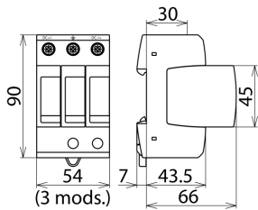
Rysunek wymiarowy DG M YPV SCI 150
