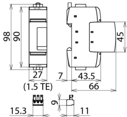
Rysunek wymiarowy DG SE DC 550 FM
