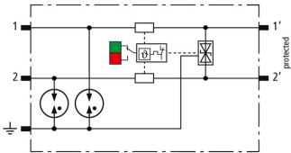
Schemat połączeń BCO CL2 BE HF 5
