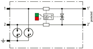
Schemat połączeń BCO CL2 BD 24
