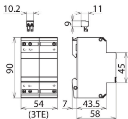
Rysunek wymiarowy BVT KKS ALD 75
