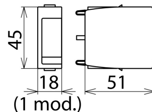
Rysunek wymiarowy DR MOD 150
