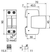
Rysunek wymiarowy DG M TN ACI 275 FM
