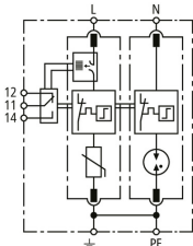
Schemat połączeń DG M TN ACI 275 FM
