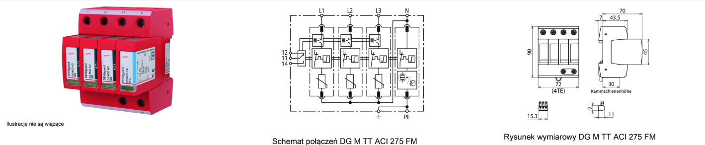
Schemat połączeń DG M TT ACI 275 FM
