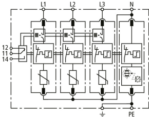
Schemat połączeń DG M TT ACI 275 FM
