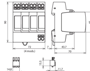
Rysunek wymiarowy DG MP TT ACI 275 FM
