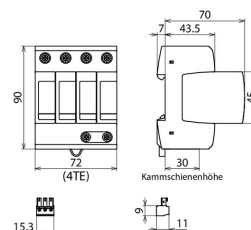
Rysunek wymiarowy DG MP TNS ACI 275 FM
