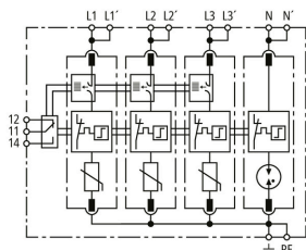
Schemat połączeń DG MP TNS ACI 275 FM
