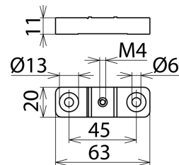
Rysunek wymiarowy ST AS SAK K
