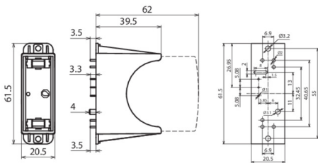
Rysunek wymiarowy DG PCB PVSCI I 500FM
