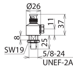
Rysunki wymiarowe DGA AG BNC
